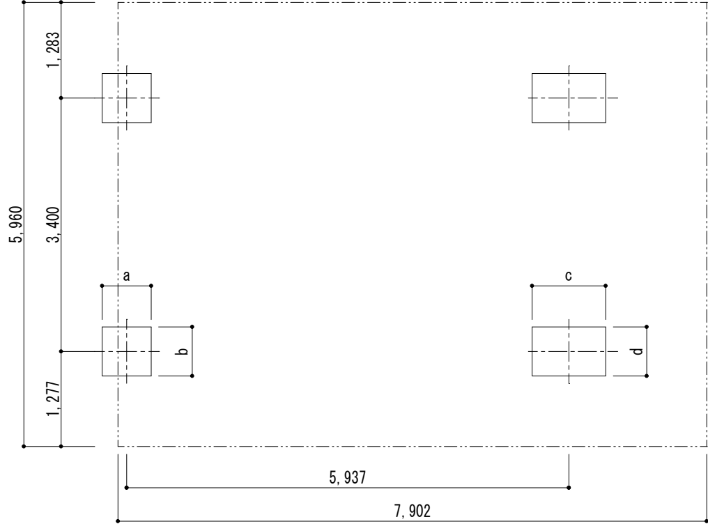
■ 基礎配置図
